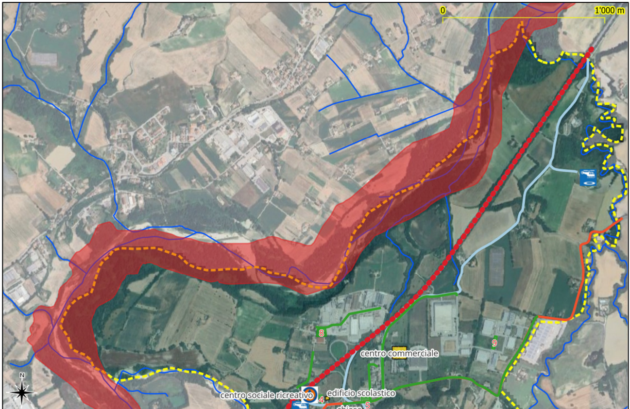
Figura 3.10 – In rosso viene restituita l’area potenzialmente interessata dal collasso della diga di San Lazzaro. Il Rischio risulta praticamente nullo per assenza di beni esposti.
